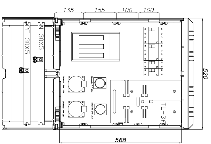
ELEWACJA ZŁĄCZA
